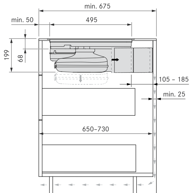
Måttskisser/ planläggning – Kolfilter – PUXU2 675 mm djup
